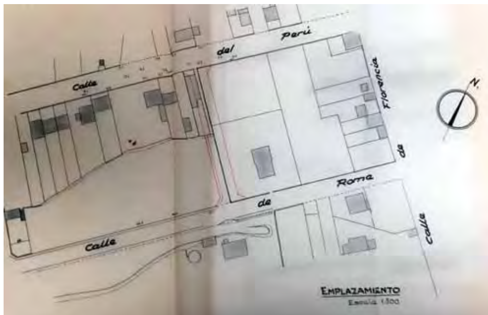
Figura 20. Plànol del projecte d'ampliació del carrer de Mozart. Es pot observar amb cert detall la parcel·lació de l'àrea com l'organització constructiva de part dels carrers Mozart, Roma, Perú i Nàpols al 1959.
