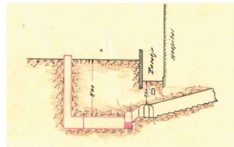
Secció del refugi antiaeri en galeria de mina de l'Hospital Municipal. (AHSCG, Caixa 281, Instàncies i certificats 1936/1938, Dictàmens 1937, núm. 281/3).
