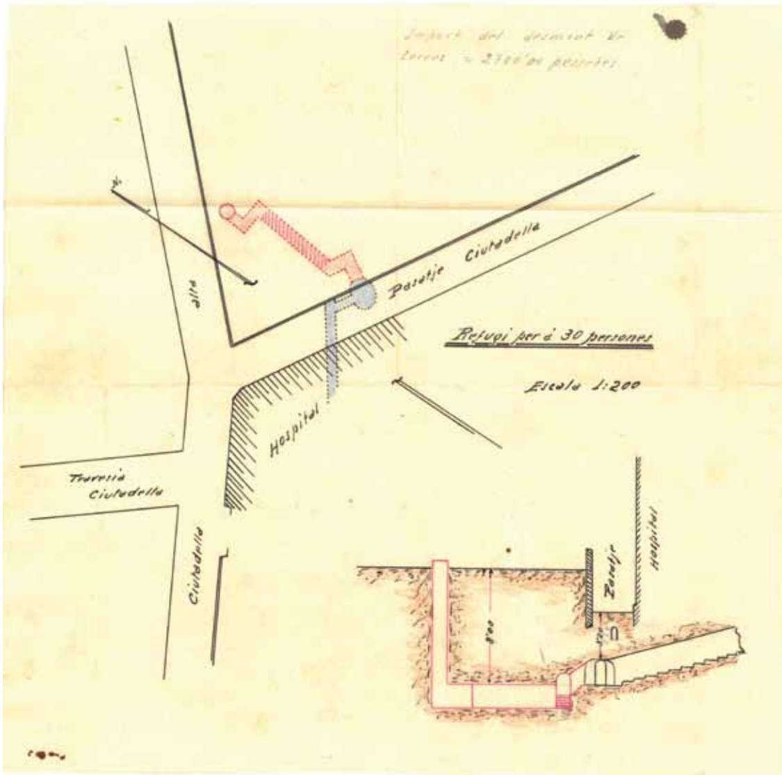
Plànol del projecte de construcció d'un refugi antiaeri a l'Hospital. (AHSCG, Caixa 281, Instàncies i certificats 1936/1938, Dictàmens 1937, núm. 281/3).
